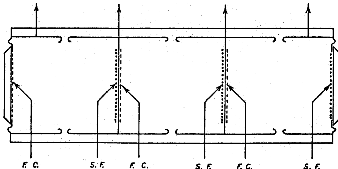
Fig. 2 - Schema di intensificatore di immagini a tre stadi in cascata.
