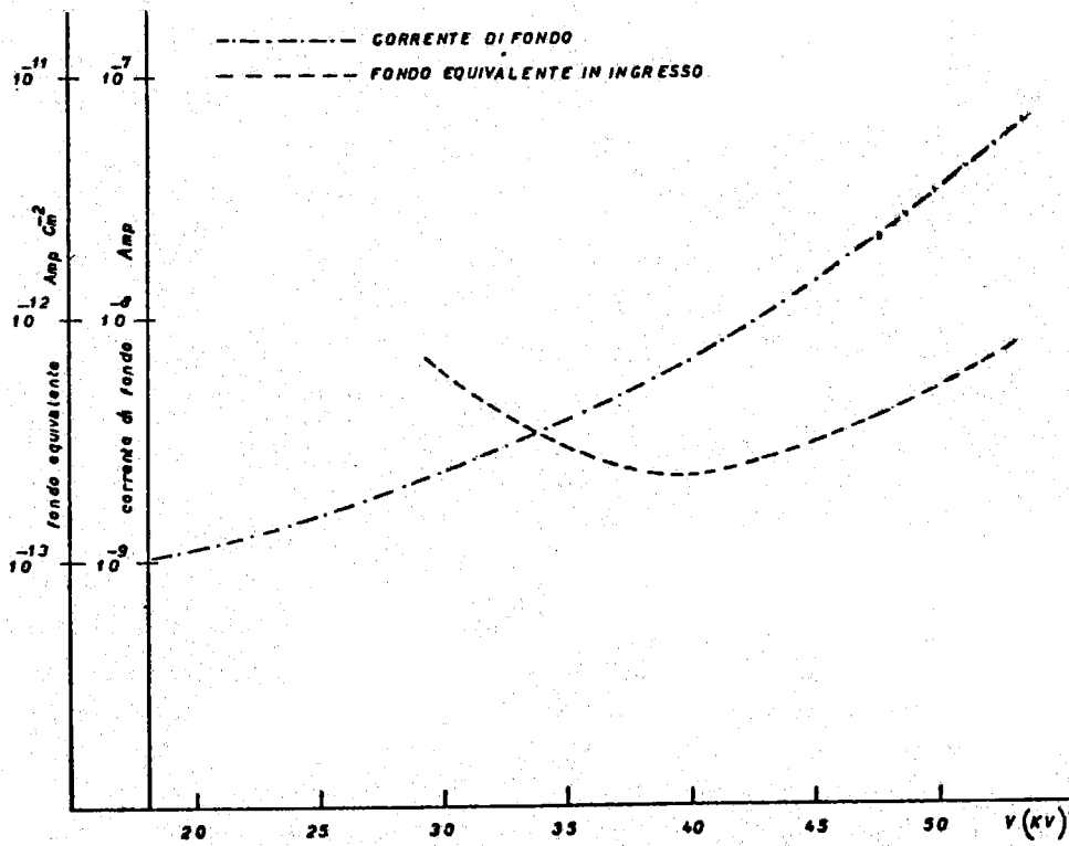
Fig. 8 - Corrente di fondo e fondo equivalente in funzione della tensione di alimentazione.
