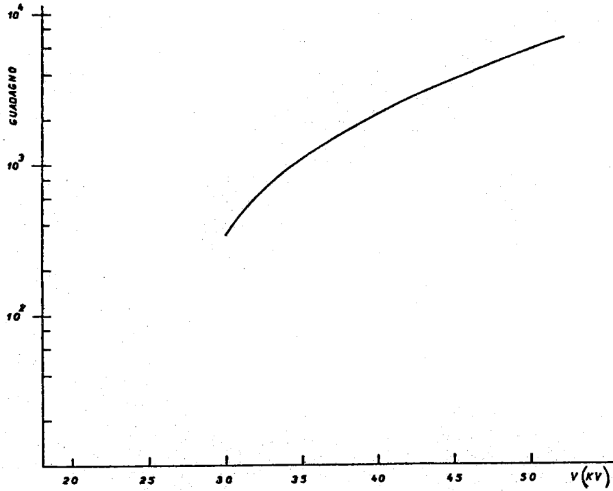
Fig. 7 - Guadagno in funzione della tensione di alimentazione.
